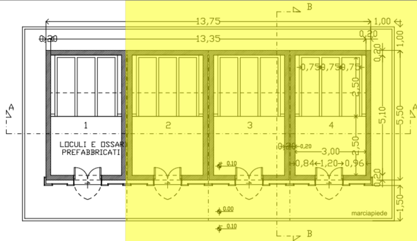
PIANTA
