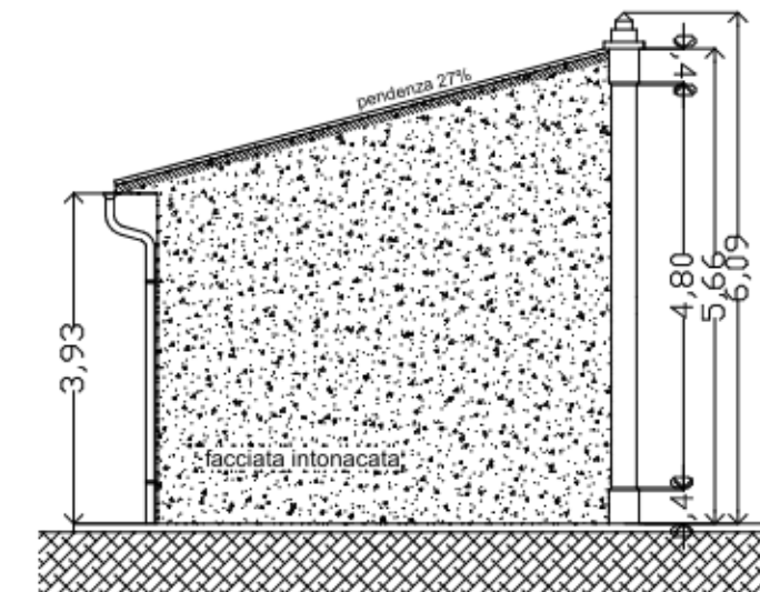
PROSPETTO LATERALE
