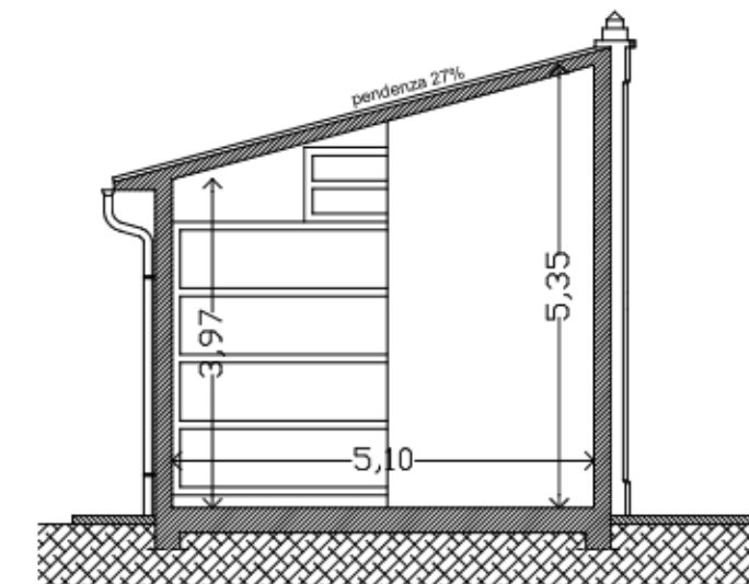
SEZIONE B-B
